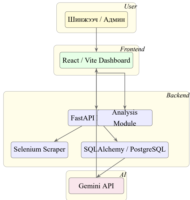
Зураг 3.2: Системийн бодит архитектурын диаграм
